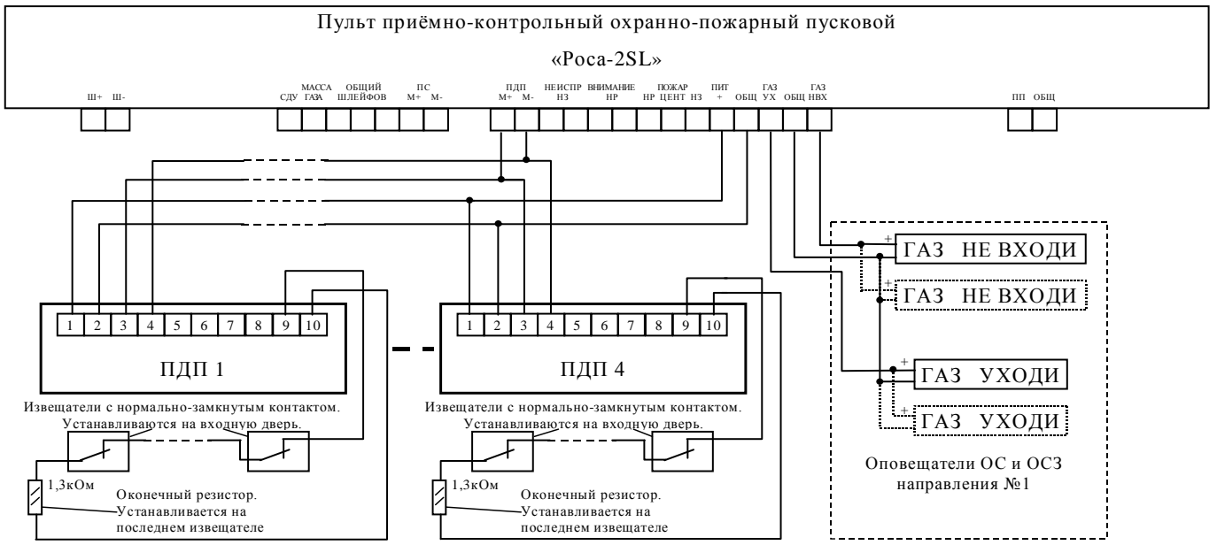
Рисунок 10. Подключение оповещателей и пульта дистанционного пуска (ПДП).
