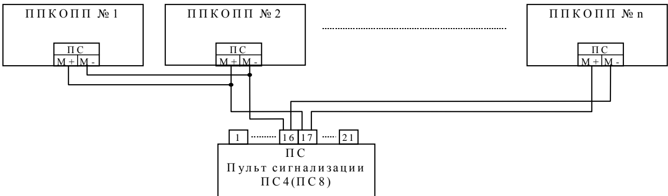
Рисунок 8. Подключение ППКOPP «Роса-2SL» к пульту сигнализации ПС8 (ПС4).
